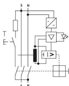
Schaltungsbeispiel Fehlerstromschutzschalter DFS 4 100-2/0,10-B NK
