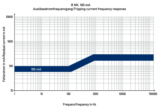
Diagramme Fehlerstromschutzschalter DFS 4 100-4/0,10-B NK V500
