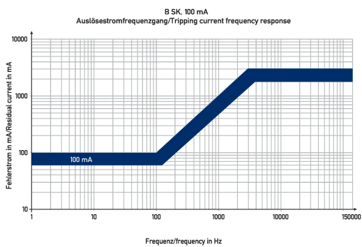
Diagramme Fehlerstromschutzschalter DFS 4 100-4/0,10-B SK V500
