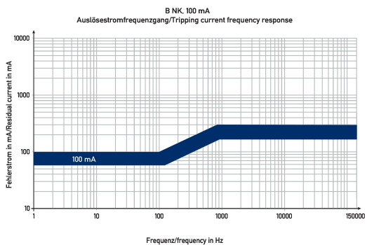
Diagramme Fehlerstromschutzschalter DFS 4 100-4/0,10-B NK
