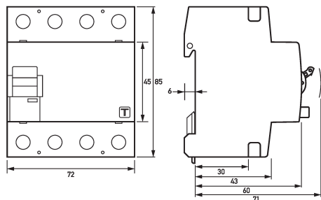
Maßzeichnung Fehlerstromschutzschalter DFS 4 100-4/0,10-B NK
