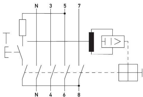
Schaltungsbeispiel Fehlerstromschutzschalter DFS 4 100-4/0,30-A
