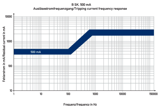
Diagramme Fehlerstromschutzschalter DFS 4 100-2/0,50-B SK
