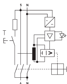
Schaltungsbeispiel Fehlerstromschutzschalter DFS 4 100-2/0,50-B SK
