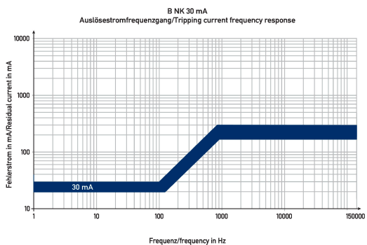
Diagramme Fehlerstromschutzschalter DFS 4 125-2/0,03-B NK
