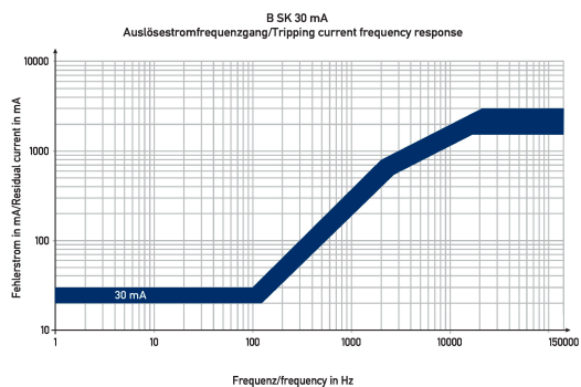
Diagramme Fehlerstromschutzschalter DFS 4 125-2/0,03-B SK
