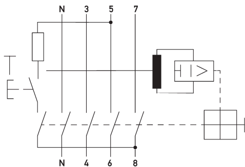
Schaltungsbeispiel Fehlerstromschutzschalter DFS 4 125-4/0,03-A V500
