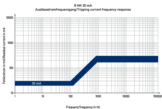
Diagramme Fehlerstromschutzschalter DFS 4 125-4/0,03-B NK V500
