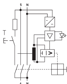
Schaltungsbeispiel Fehlerstromschutzschalter DFS 4 125-2/0,10-B+
