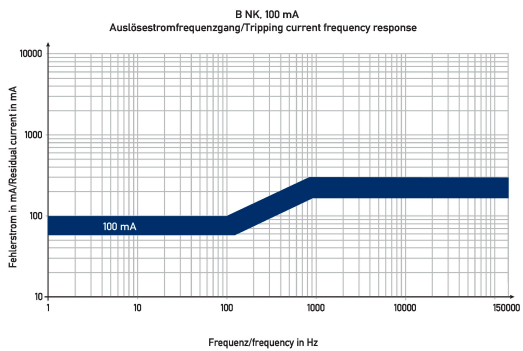
Diagramme Fehlerstromschutzschalter DFS 4 125-2/0,10-B NK
