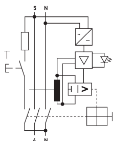
Schaltungsbeispiel Fehlerstromschutzschalter DFS 4 125-2/0,10-B NK
