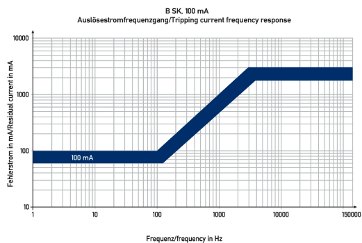
Diagramme Fehlerstromschutzschalter DFS 4 125-2/0,10-B SK
