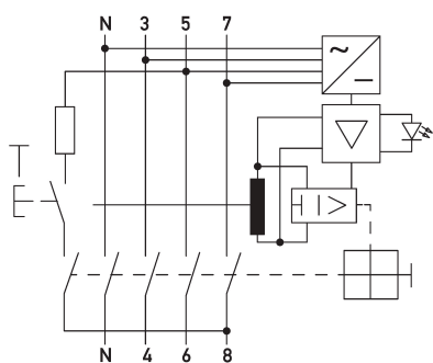
Schaltungsbeispiel Fehlerstromschutzschalter DFS 4 125-4/0,10-B+
