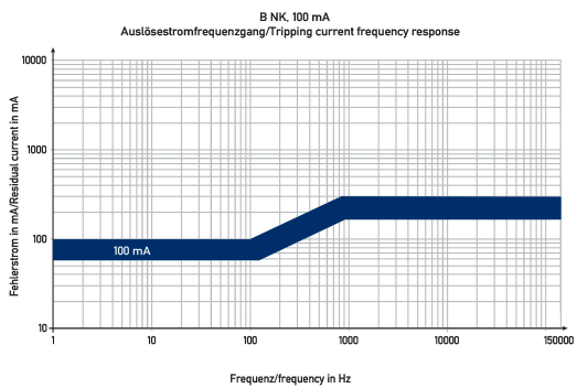
Diagramme Fehlerstromschutzschalter DFS 4 125-4/0,10-B NK
