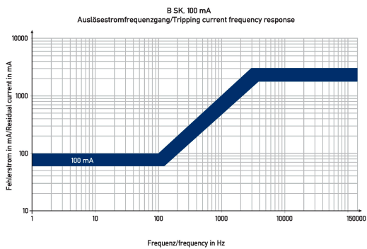
Diagramme Fehlerstromschutzschalter DFS 4 125-4/0,10-B SK
