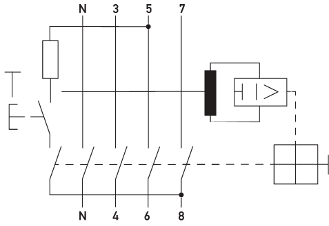
Schaltungsbeispiel Fehlerstromschutzschalter DFS 4 125-4/0,30-A V500
