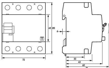
Maßzeichnung Fehlerstromschutzschalter DFS 4 125-4/0,30-A V500
