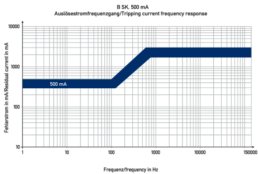
Diagramme Fehlerstromschutzschalter DFS 4 125-2/0,50-B SK
