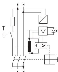
Schaltungsbeispiel Fehlerstromschutzschalter DFS 4 125-2/0,50-B SK
