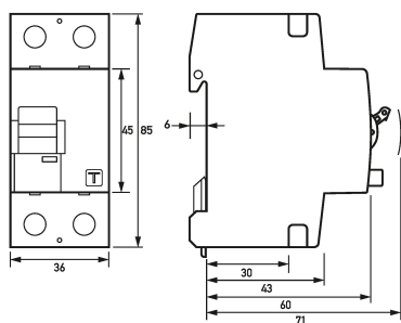
Maßzeichnung Fehlerstromschutzschalter DFS 2 100-2/0,03-F
