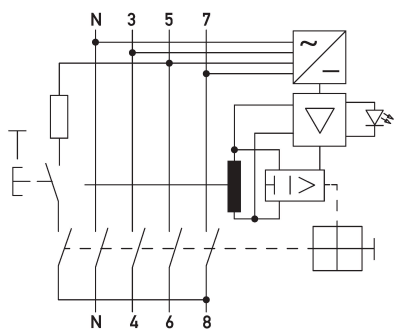
Schaltungsbeispiel Fehlerstromschutzschalter DFS 4 080-4/0,30-B+ HD
