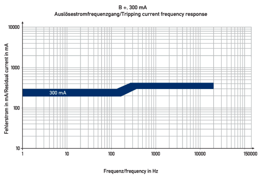
Diagramme Fehlerstromschutzschalter DFS 4 080-4/0,30-B+ HD
