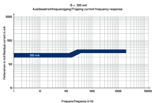
Diagramme Fehlerstromschutzschalter DFS 4 025-4/0,30-B+ HD
