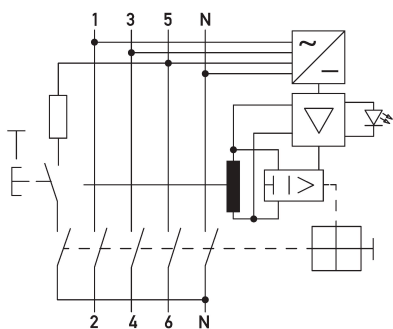
Schaltungsbeispiel Fehlerstromschutzschalter DFS 4 040-4/0,30-B SK R
