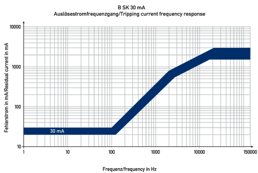
Diagramme Fehlerstromschutzschalter DFS 4 080-4/0,03-B SK HD
