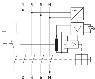
Schaltungsbeispiel Fehlerstromschutzschalter DFS 4 063-4/0,03-B SK R HD
