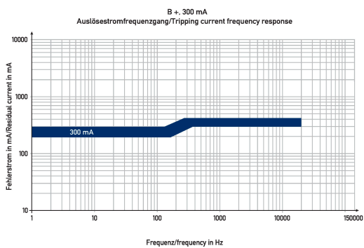
Diagramme Fehlerstromschutzschalter DFS 4 040-4/0,30-B+ HD
