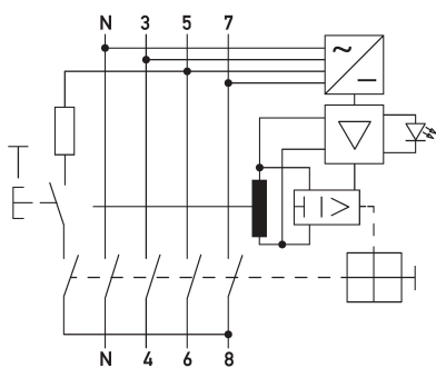
Schaltungsbeispiel Fehlerstromschutzschalter DFS 4 100-4/0,30-B NK HD
