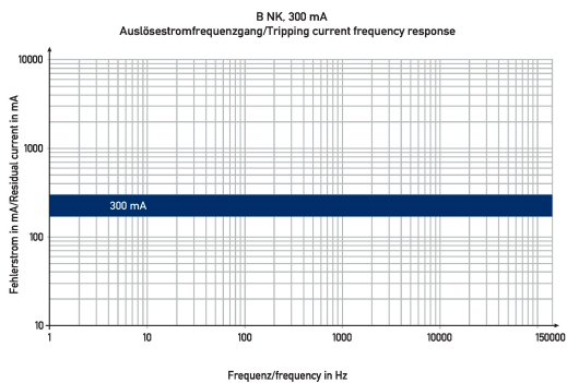
Diagramme Fehlerstromschutzschalter DFS 4 100-4/0,30-B NK HD
