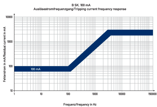
Diagramme Fehlerstromschutzschalter DFS 4 040-4/0,10-B SK HD
