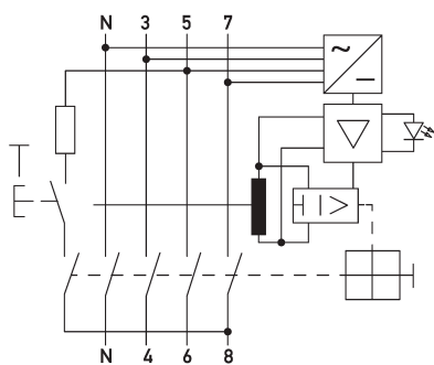
Schaltungsbeispiel Fehlerstromschutzschalter DFS 4 125-4/0,30-B NK HD
