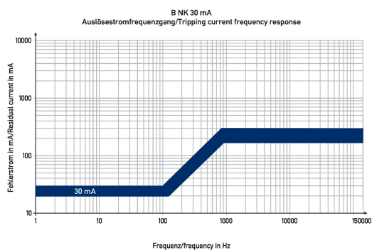
Diagramme Fehlerstromschutzschalter DFS 4 063-4/0,03-B NK HD
