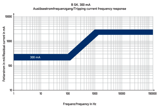
Diagramme Fehlerstromschutzschalter DFS 4 080-4/0,30-B SK HD
