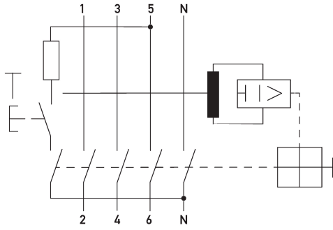
Anschlusschema
