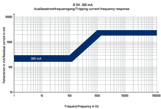
Diagramme Fehlerstromschutzschalter DFS 2 080-2/0,30-B SK
