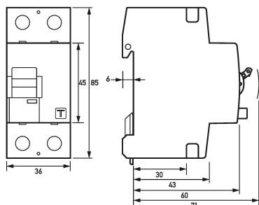
Maßzeichnung Fehlerstromschutzschalter DFS 2 080-2/0,30-B NK
