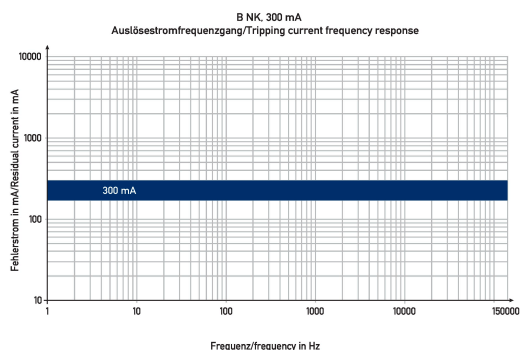
Diagramme Fehlerstromschutzschalter DFS 2 080-2/0,30-B NK
