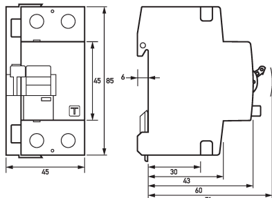
Maßzeichnung Fehlerstromschutzschalter DFS 2 025-2/0,10-A FT
