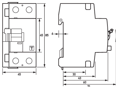
Maßzeichnung Fehlerstromschutzschalter DFS 2 025-2/0,10-A FT
