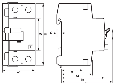
Maßzeichnung Fehlerstromschutzschalter DFS 2 025-2/0,50-A FT
