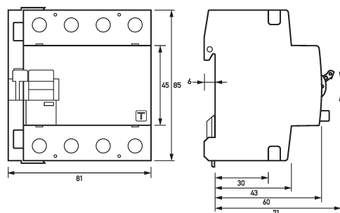
Maßzeichnung Fehlerstromschutzschalter DFS 4 063-4/0,10-A FT
