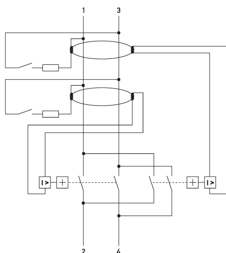
Schaltungsbeispiel Fehlerstromschutzschalter DFS 2 080-2/0,03-A KV Twin
