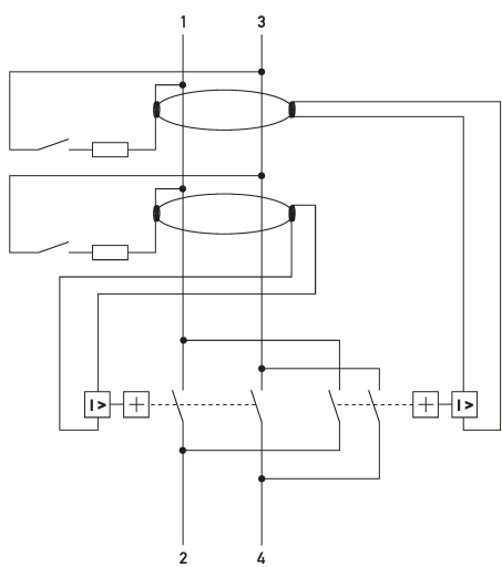
Anschlusschema
