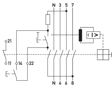
Anschlusschema
