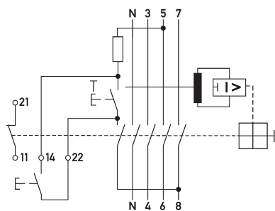
Schaltungsbeispiel Fehlerstromschutzschalter DFS 4 125-4/0,03-A FT
