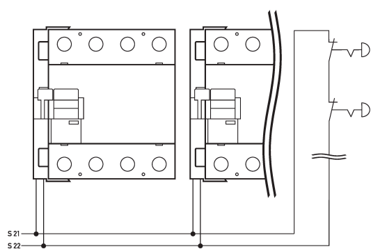
Schaltungsbeispiel Fehlerstromschutzschalter DFS 4 063-4/0,03-A NA
