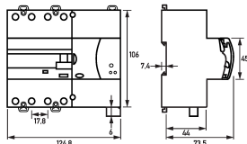
Maßzeichnung Gruppenansicht
