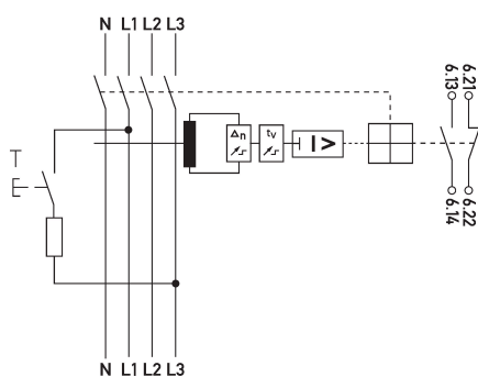
Schaltungsbeispiel Leistungsschalter mit Fehlerstromschutz DFL 8 200-4/X-A
