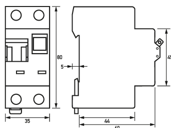
Maßzeichnung FI-/LS-Kombinationen DRCBO 3 B32/0,03/1N-A KV
