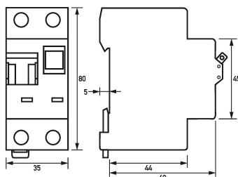
Maßzeichnung FI-/LS-Kombinationen DRCBO 3 B25/0,03/1N-F
