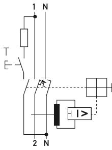
Schaltungsbeispiel FI-/LS-Kombinationen DRCBO 3 C40/0,03/1N-F
