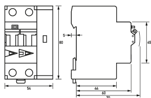
Maßzeichnung Fehlerlichtbogen-Schutzeinrichtungen DAFDD 1 C40/0,03/2-A
