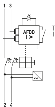
Schaltungsbeispiel Fehlerlichtbogen-Schutzeinrichtungen DAFDD 1 C40/0,03/2-A
