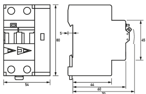
Maßzeichnung Fehlerlichtbogen-Schutzeinrichtungen DAFDD 1 C25/0,03/2-A
