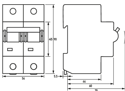
Maßzeichnung Gruppenansicht
