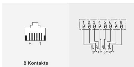
8 Kontakte
